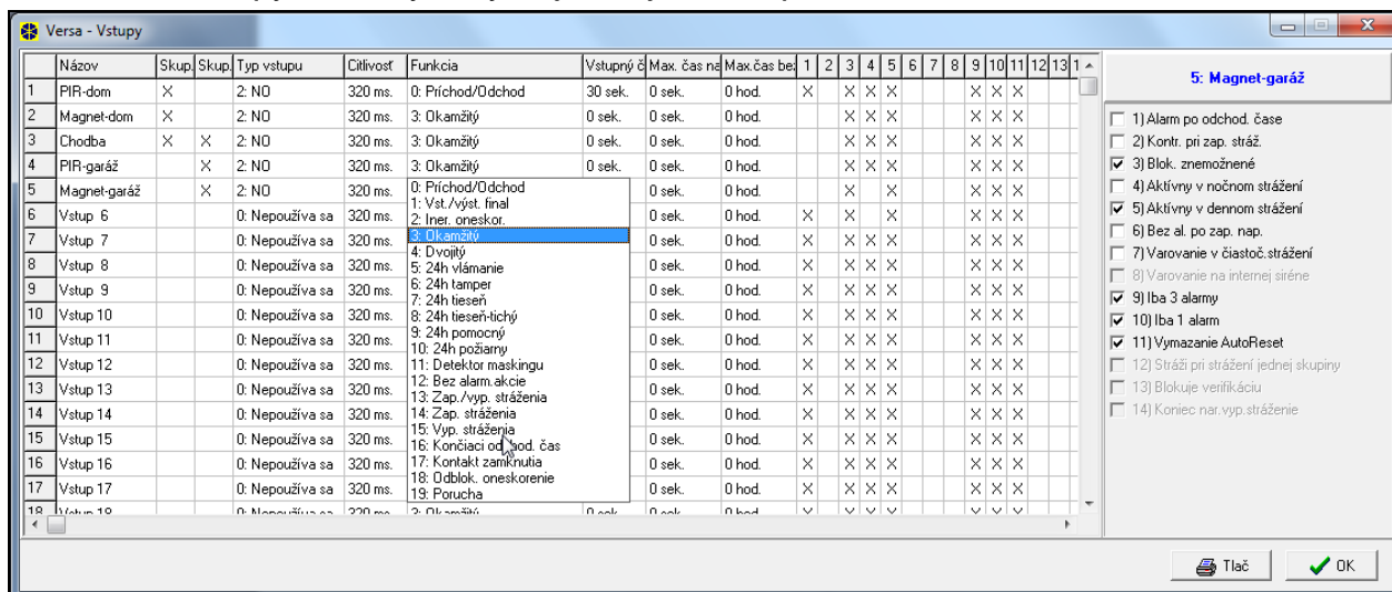
Obr. 8. Okno „Versa – Vstupy” v programe DLOADX.
