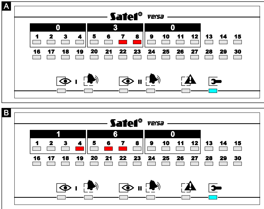
Obr. 1. Príklady zobrazenia desiatkových hodnôt (DEC) pomocou LED-iek na LED klávesnici. V príklade A je naprogramovaná hodnota 30 (030), a v príklade B – 160.
