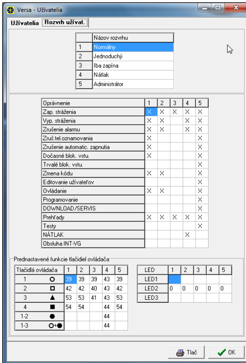
Obr. 19. Programovanie schém užívateľov v okne „Versa – Uživatelia” v programe DLOADX (príklad nastavenia).
