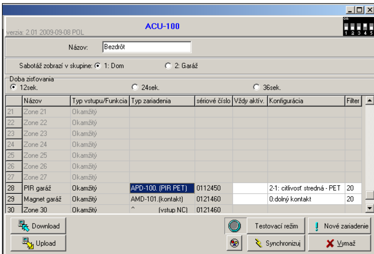
Obr. 14. Programovanie nastavení kontroléra bezdrôtového systému a bezdrôtových zariadení v programe DLOADX (príklad konfigurácie).
