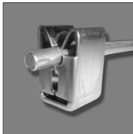
Spannhalter SP ( držiak - klip )
