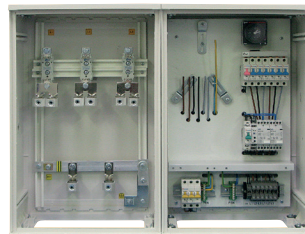
RVO 2 + 100 / NKE 8P FH06
