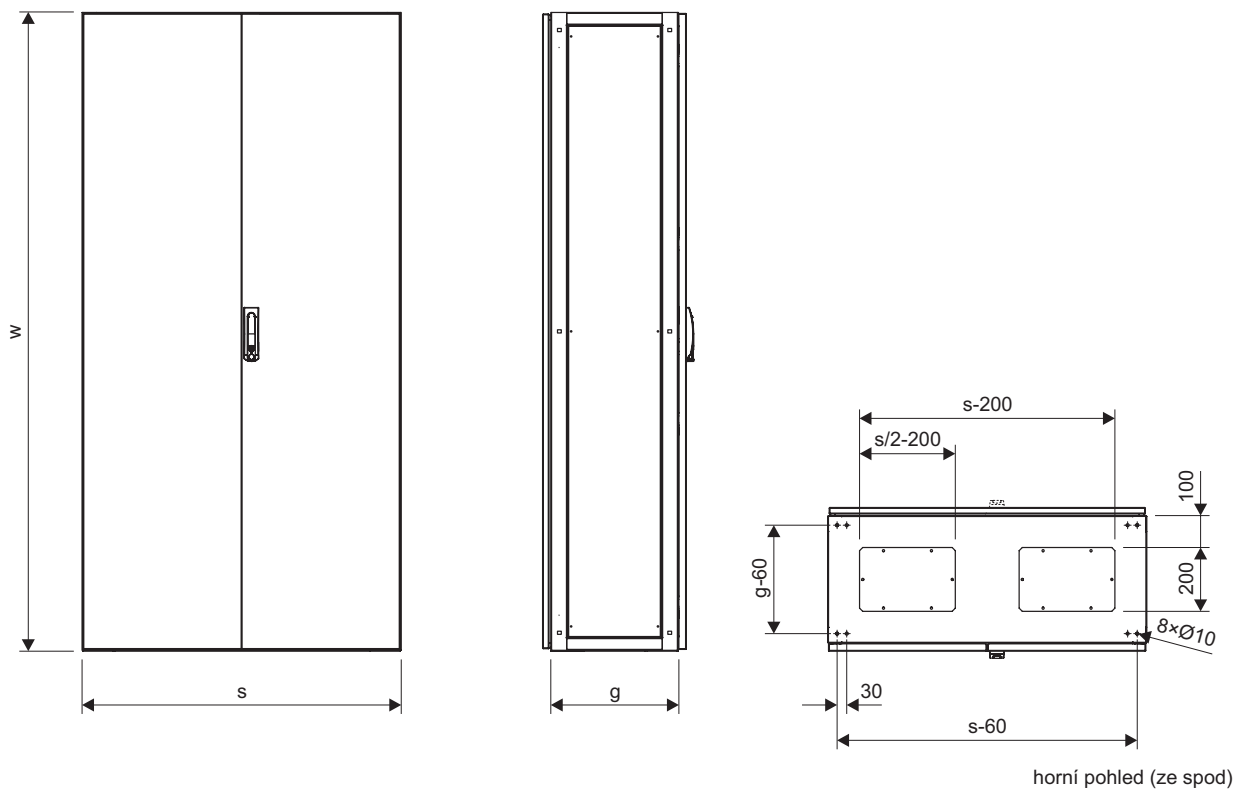
Skříně 2-dveřová:
