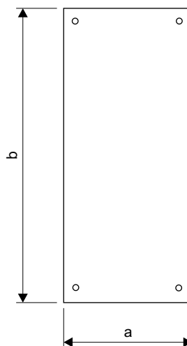
Montážní deska
