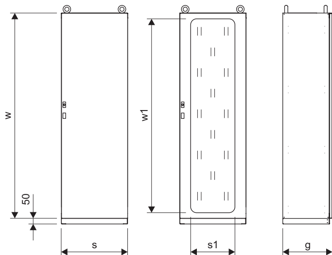
Skříň OWW 1 - dveřová
