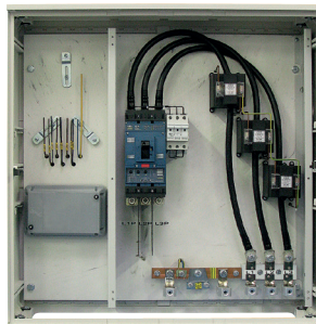
NR 111 / NVD 7
