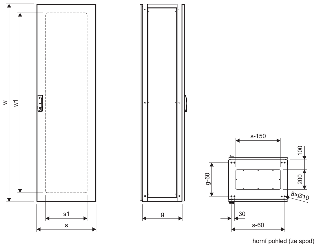
Obrázky Skříně 1-dveřová:
