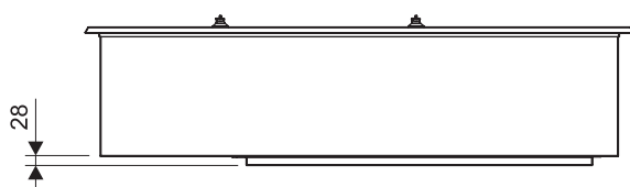
skříňka SWA ... - zadní pohled
