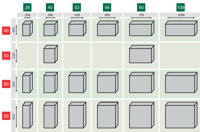
Přehledová tabulka skříní S s hloubkou 240 mm
